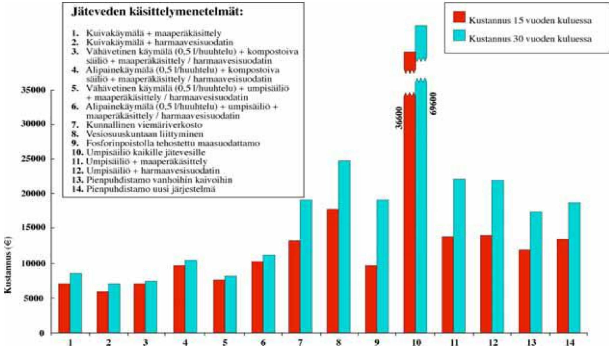
Kuva 3. Eri jätevesijärjestelmien kustannukset 15 ja 30 vuoden ajanjaksolla. Kustannuksissa ovat mukana sekä investointi-, käyttö- että mahdolliset uusimiskustannukset.
